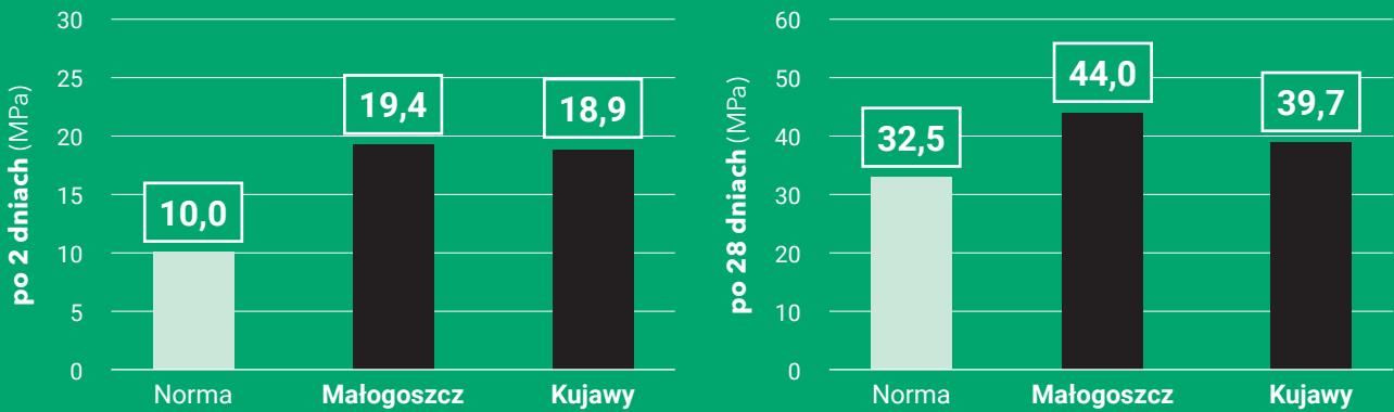
Wytrzymałość na ściskanie badana zgodnie z PN-EN 196-1
