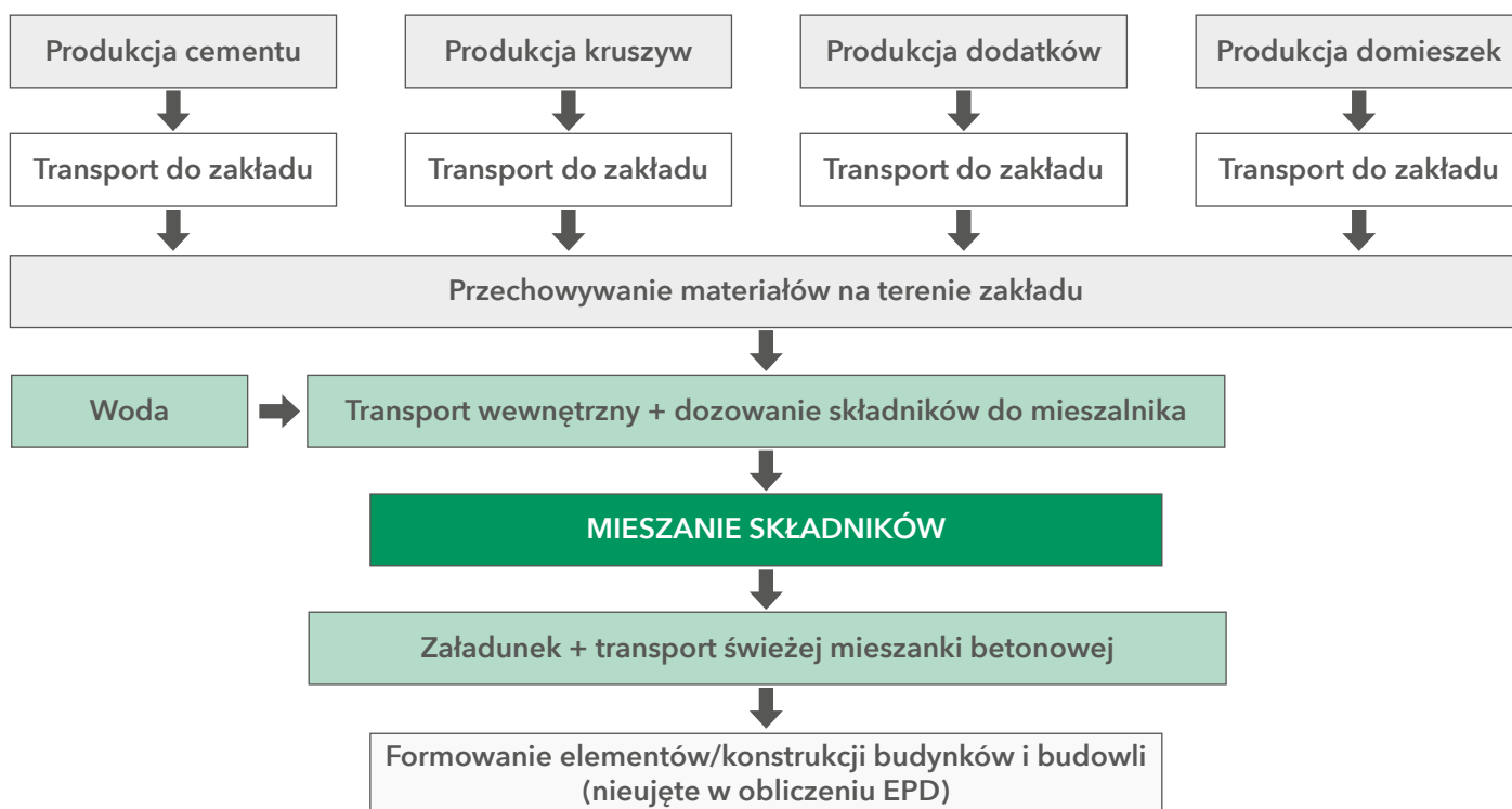
Rysunek 2. Produkcja mieszanki betonowej - nakłady i procesy systemu produkcyjnego
