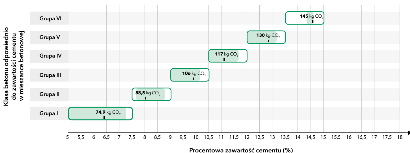
Rysunek 1. Podział na grupy w zależności od zawartości cementu w recepturze mieszanki betonowej
