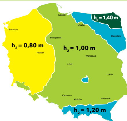
Rys. 1. Strefy przemarzania gruntu w Polsce. Źródło: GIG
