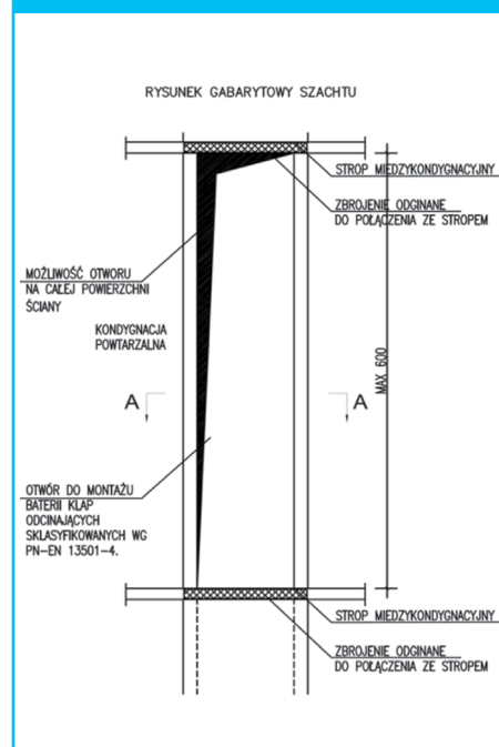
rys. 3. przykŁad realizacji szachtu wraz z otworami na kondygnacji powtarzalnej
