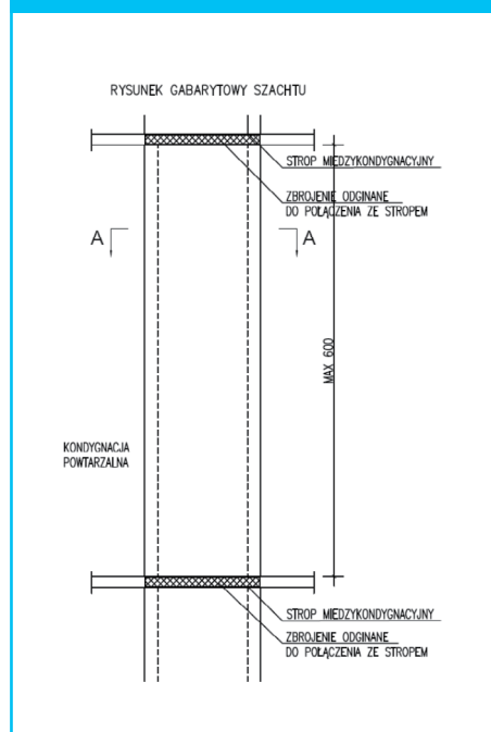
rys. 2. przykŁad realizacji szachtu bez otworów
