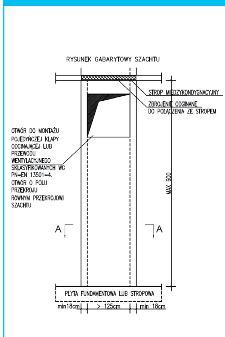
rys. 1. przykŁad realizacji szachtu z otworami na kondygnacji
