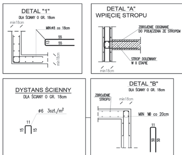
RYS. 6. RYSUNKI PRZYKŁADOWYCH DETALI
