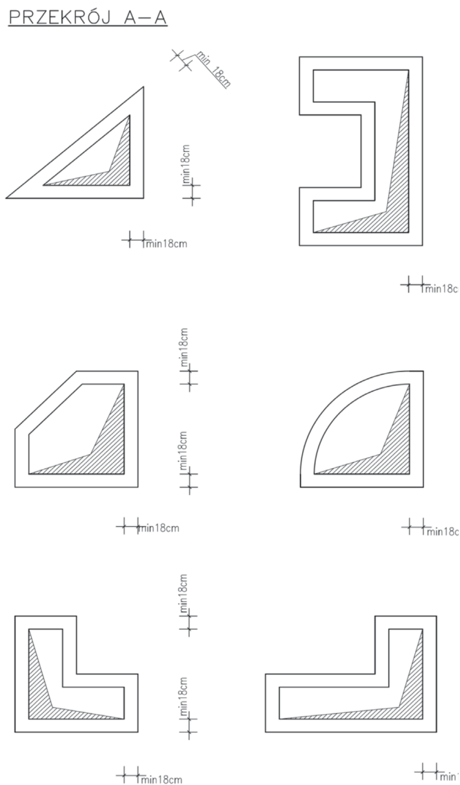
RYS. 7. PRZEKRÓJ PRZESZACHT NIEREGULARNY - PRZYKŁADY
