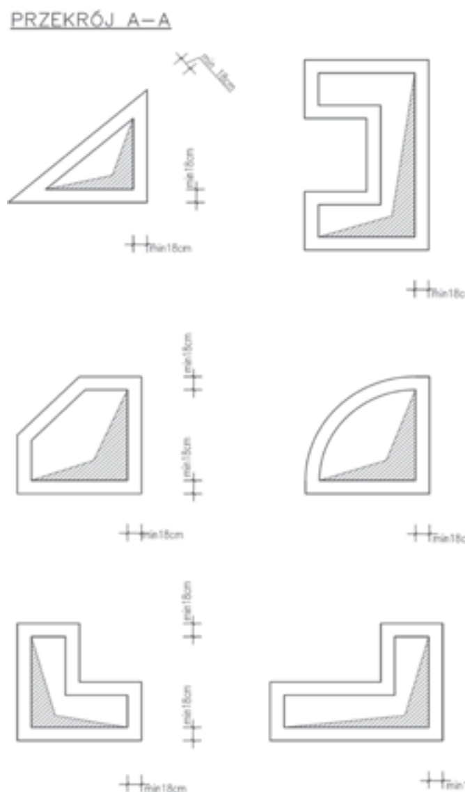
rys. 7. przekrój przez szacht nieregularny - przykłady
