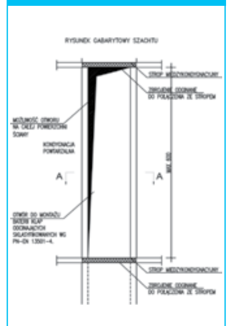
RYS. 3. PRZYKŁAD REALIZACJI SZACHTU WRAZ Z OTWORAMI NA KONDYGNACJI POWTARZALNEJ
